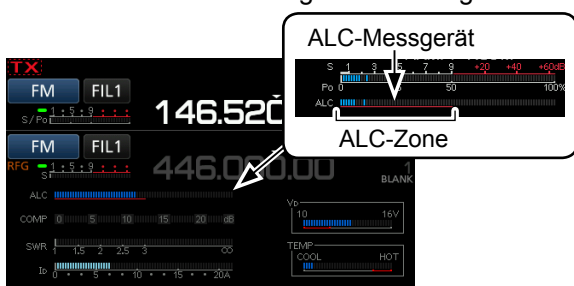
Multifunktionsmessgerät
